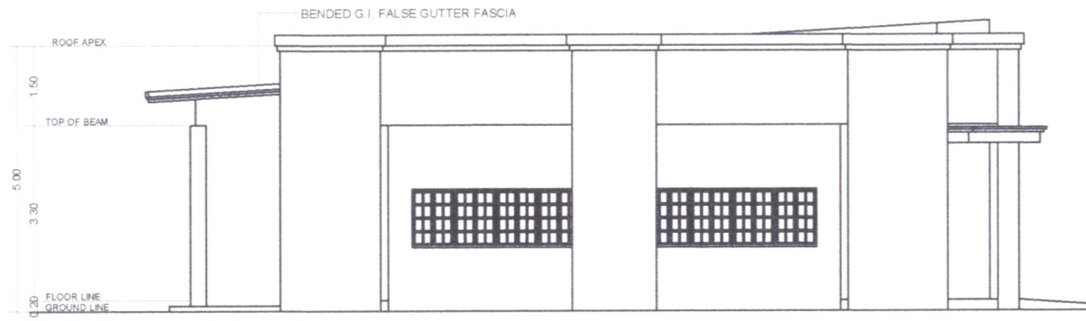
LEFT-SIDE ELEVATION SCALE: 1:120MTS
